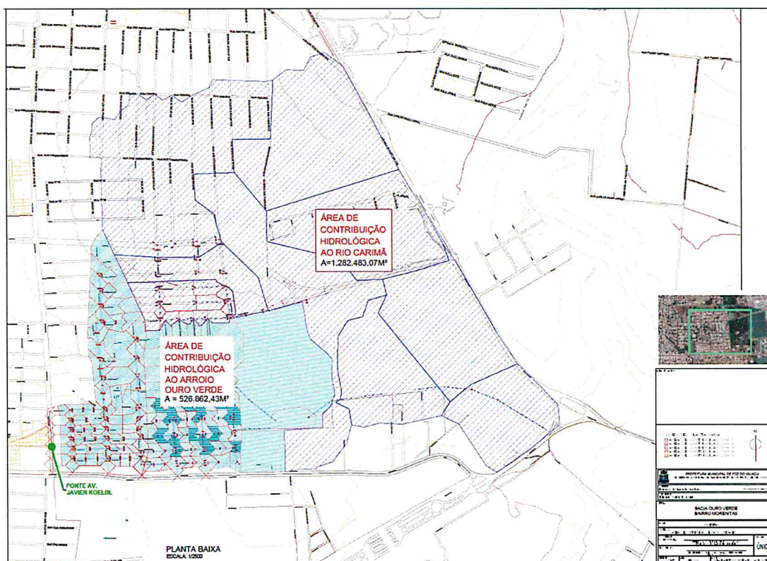
Figura 1: Área de Intervenção Projetos do Arroio Ouro Verde
