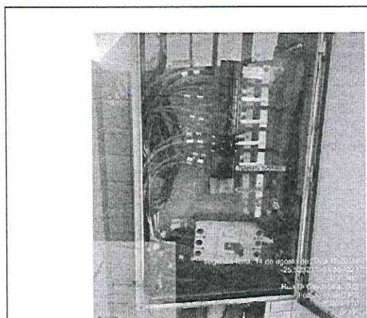
ITEM 5.3.2 – DISJUNTOR TRIFÁSICO 300A
