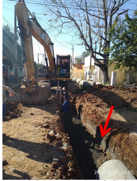
Imagem 3 – Escavação e colocação de brita – Rua Rômulo Carbone
