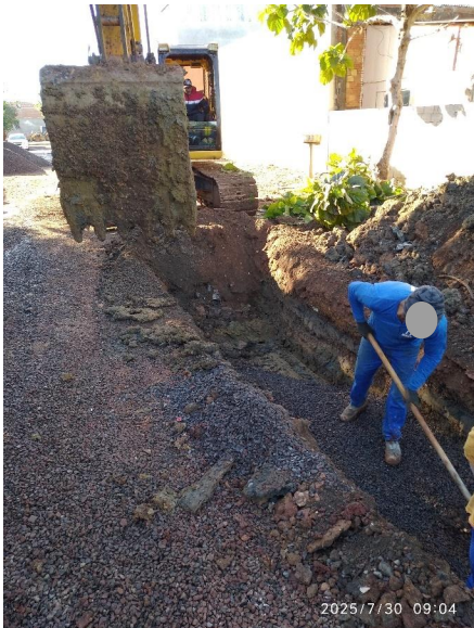
Imagem 17 – Abertura das valas e espalhamento do colchão de brita
